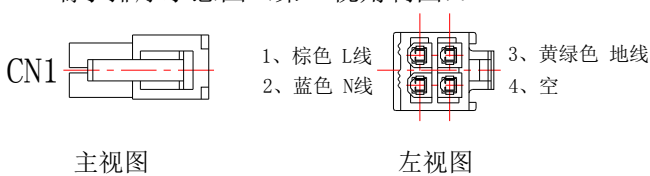
端子排序示意图 (第一视角制图):
