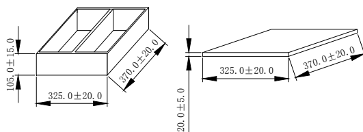
珍珠棉板
