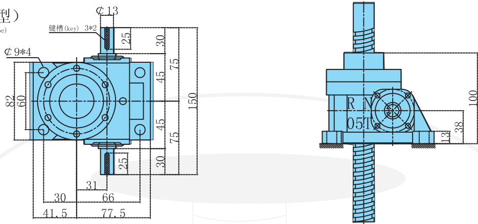
②直接式 (Direct type) 单入 (single input) 右侧 (flanged right side)
