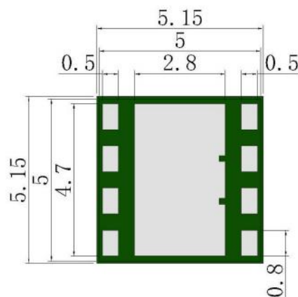
背面图
