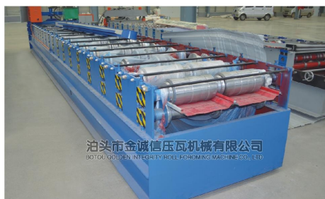
JCX820隐藏式彩钢瓦成型机（前切刀） Joint-hidden Type Forming Machine(Pre Cut)
