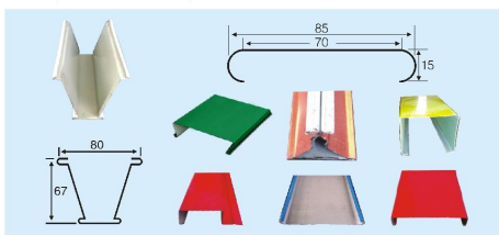
新型灯箱广告扣板机 Lamp house roll forming machine
