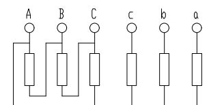
Dyn11
