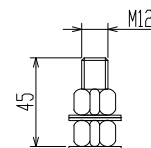
HV terminal
