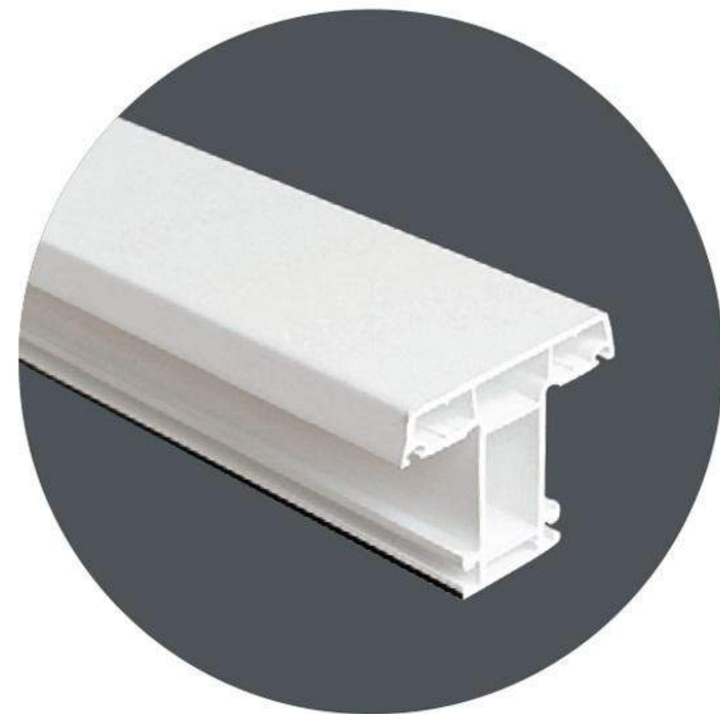
60B 中挺 60B Frame mullion
