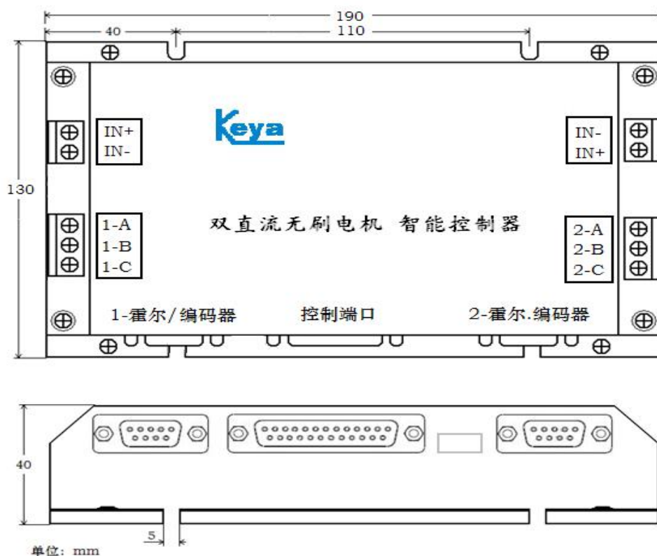
外形尺寸图
