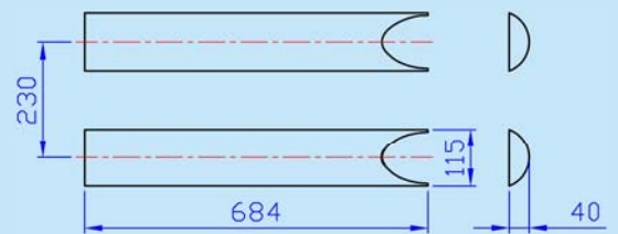
下模平面示意圖 Lower mould diagram
