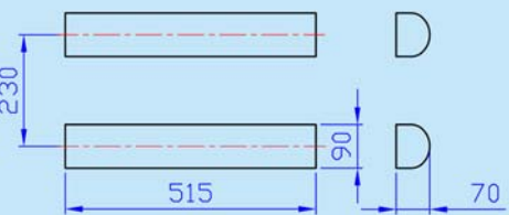
下模平面示意圖 Lower mould diagram
