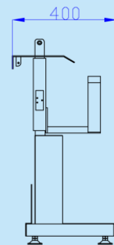
機身尺寸 Machine Size Diagram
