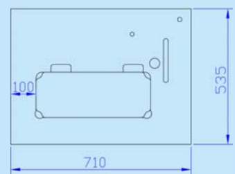
短檯板尺寸 Short Table Dimensions
