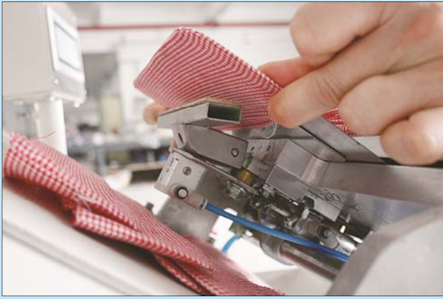
自動底夾，防止操作時袖口移位 Automatic bottom clamp for avoiding cuff shift
