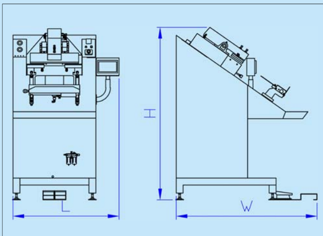
機身外形尺寸圖 Machine external dimensions diagram
