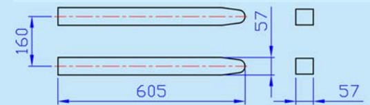
下模平面示意圖 Lower mould diagram
