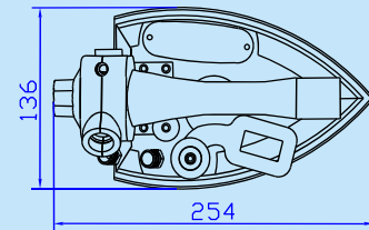
熨斗尺寸簡圖 Iron Dimensions Diagram(mm)
