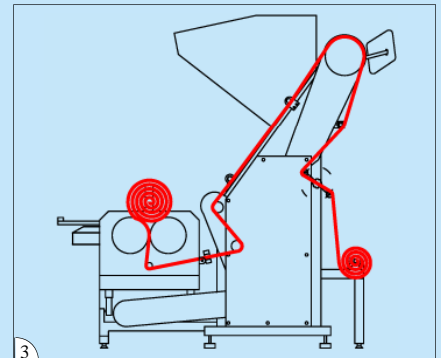
上布示意圖 Fabric routing diagram
