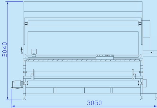
機身尺寸及穿布示意圖 Machine Size & Cloth Travel Diagram
