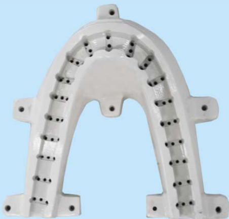
K款下模 Lower mould Type K 編號：M13050110
