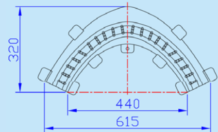
J款下模 Lower mould Type J 編號：M13050109
