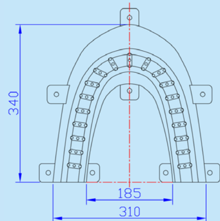
K款下模 Lower mould Type K 編號：M13050110
