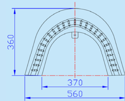
C款下模 (標準跟機模) Lower mould Type C (Standard) 編號：M13050103-1
