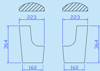
下模尺寸簡圖 Size of Lower Mould
