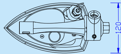
熨斗尺寸簡圖 Iron Dimensions Diagram (mm)
