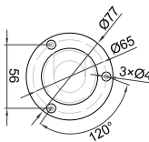
底座安装孔
