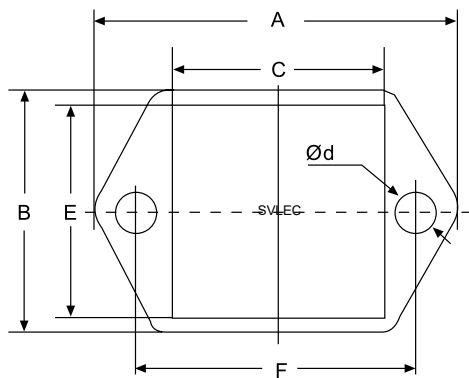
H3A 开孔底座 housing
