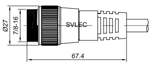
插针 Male 直出 Straight
