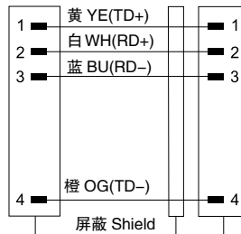
2x2x22AWG & 2x2x24AWG
