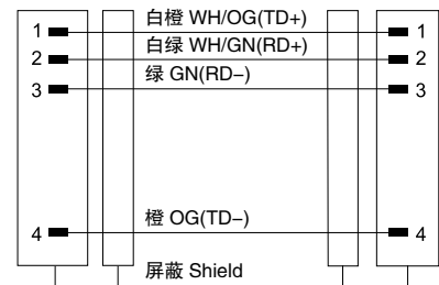
2x2x26AWG
