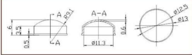
二维图纸 2Ddrawing
