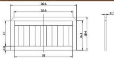
二维图纸 2Ddrawing
