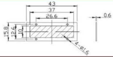
二维图纸 2Ddrawing
