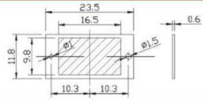
二维图纸 2Ddrawing
