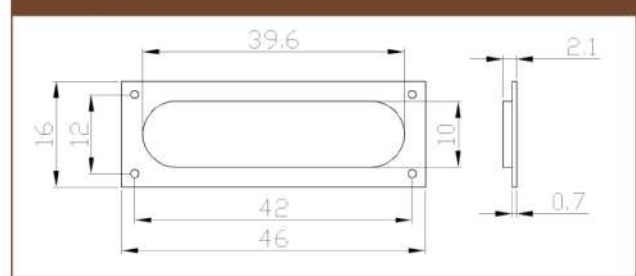
二维图纸 2Ddrawing
