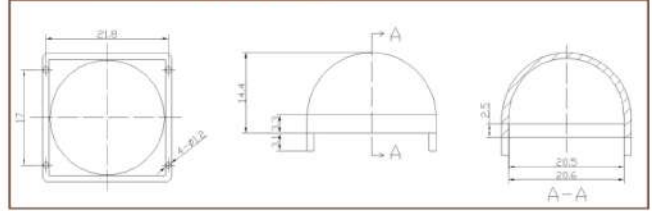
二维图纸 2Ddrawing
