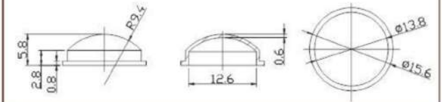
二维图纸 2Ddrawing
