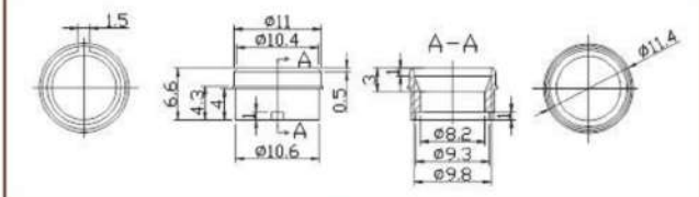
二维图纸 2Ddrawing
