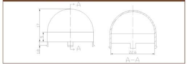
二维图纸 2Ddrawing
