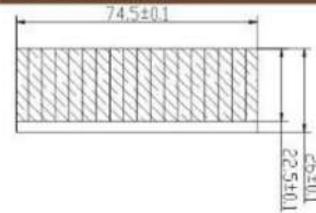
二维图纸 2Ddrawing
