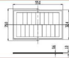
二维图纸 2Ddrawing
