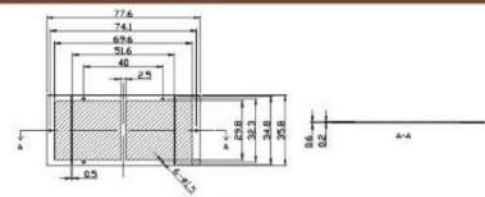
二维图纸 2Ddrawing
