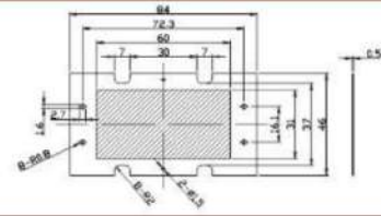
二维图纸 2Ddrawing
