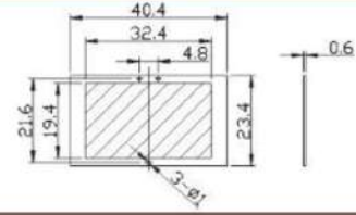
二维图纸 2Ddrawing
