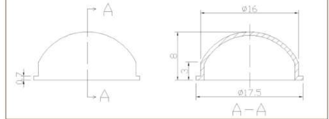
二维图纸 2Ddrawing
