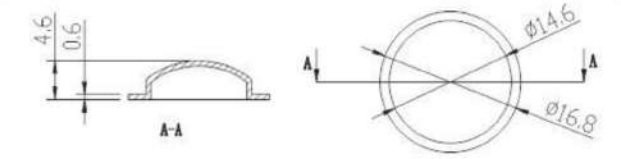
二维图纸 2Ddrawing
