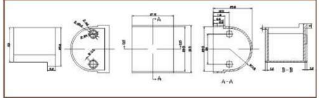
二维图纸 2Ddrawing
