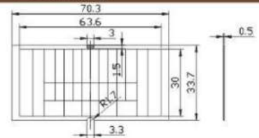
二维图纸 2Ddrawing
