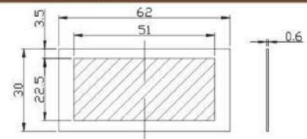
二维图纸 2Ddrawing
