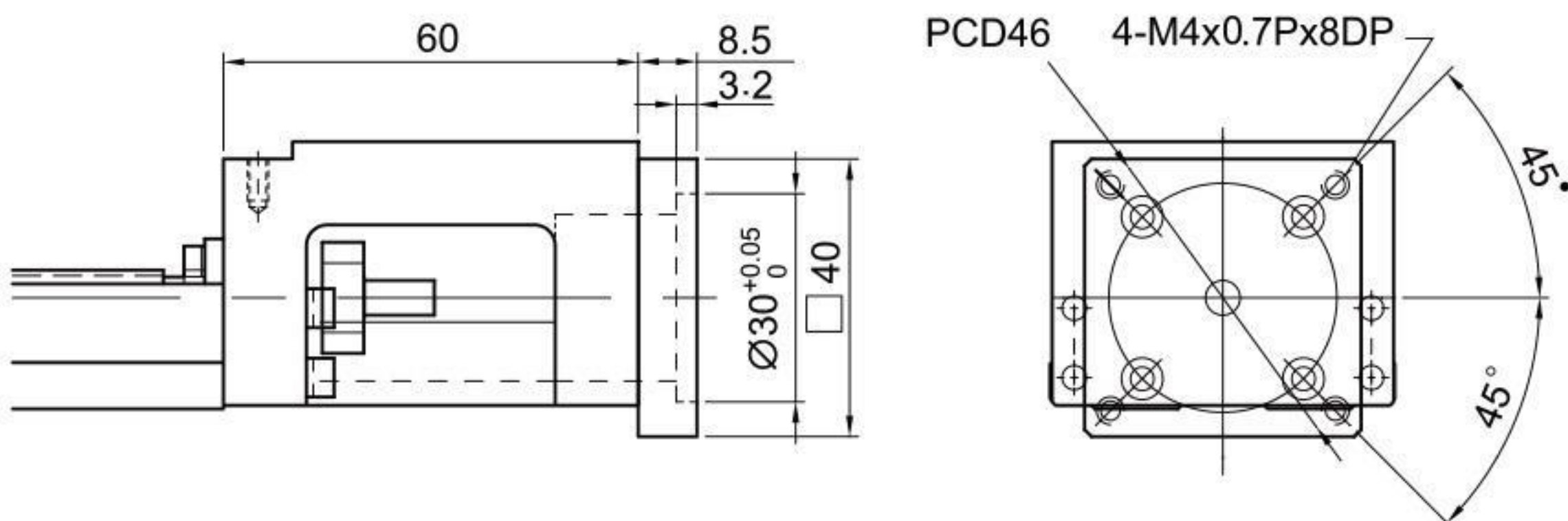
Motor Adaptor Flange F1
