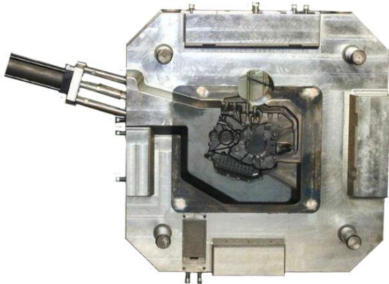
Automobile Steering Gear Diverter Die Casting Mould 汽车转向机转向器压铸模具
