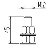
HV terminal
