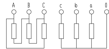
Dyn11
