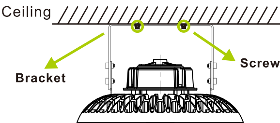
2.Bracket type
