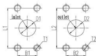
Inlet/Outlet Flange Combination - 进出油口法兰连接 ( #型 ■ )
