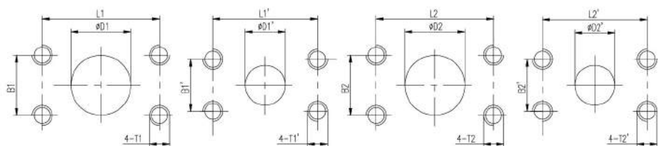
Double Pump Inlet/Outlet Flange Combination 双联泵油口法兰组合
