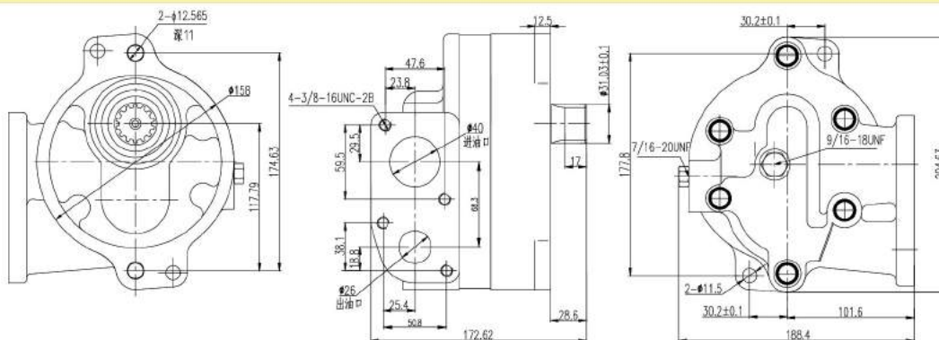
2P9239 Installation Dimensions - 2P9239 齿轮泵外型图
