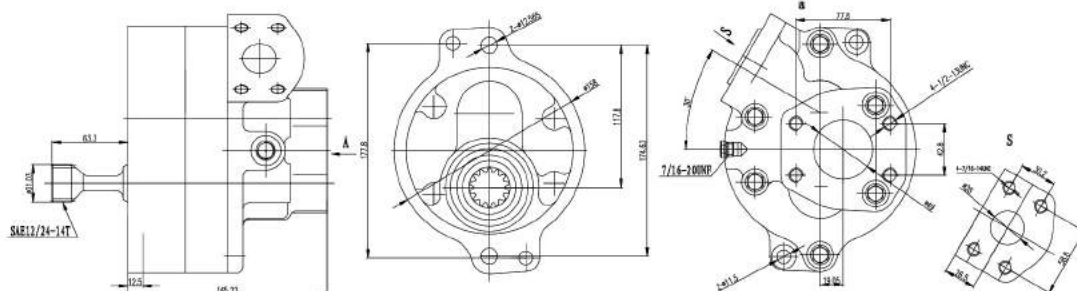
2P9239 Installation Dimensions - 2P9239 齿轮泵外型图
