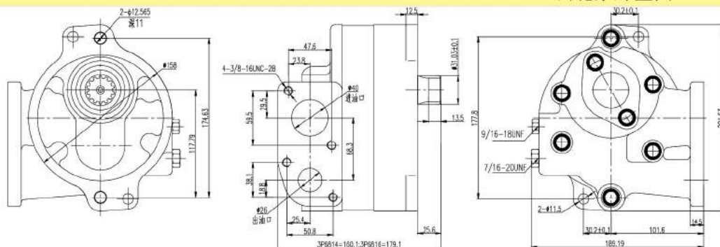
3P6816 / 3P6814 Installation Dimensions - 3P6816 / 3P6814 齿轮泵外型图
