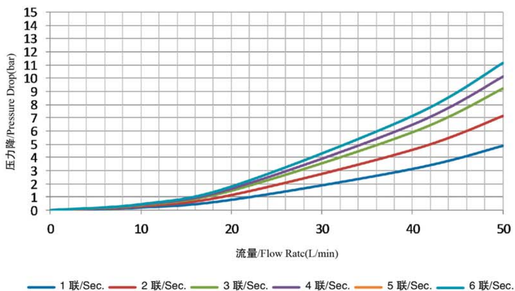
Neutral position (P to T) 中位时, 进口口到油箱的压力降 (P to T)
