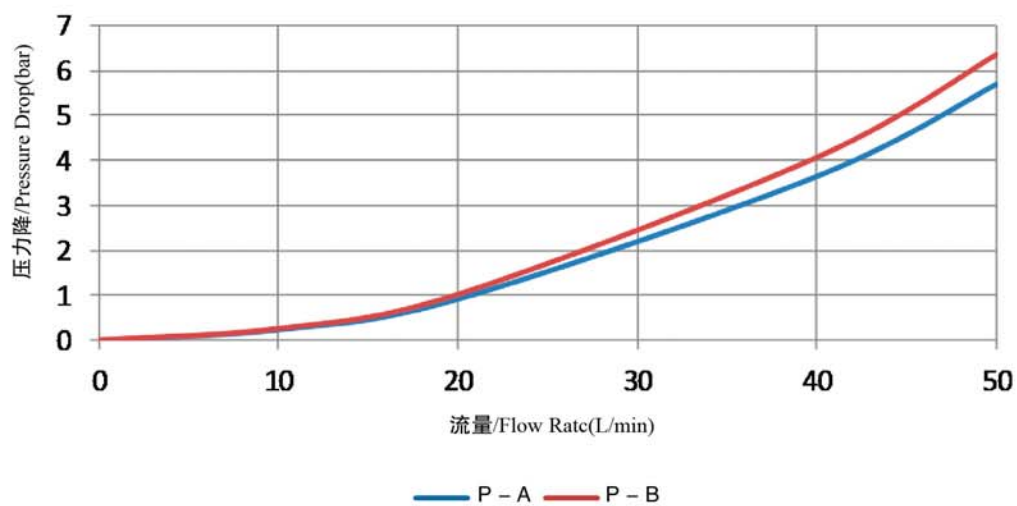
Inlet to Work Port 进油口到工作油口的压力降
