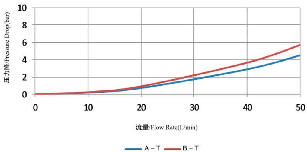
Work Port to Tank 工作油口到油箱压力降
