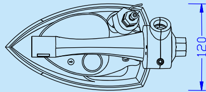
熨鬥尺寸簡圖 Iron Dimensions Diagram (mm)
