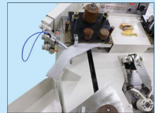
機械夾自動收料 Automatic clamp for collar stacking automatically
