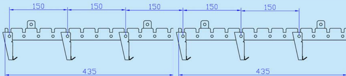
標準掛距 Standard hanging spacing
