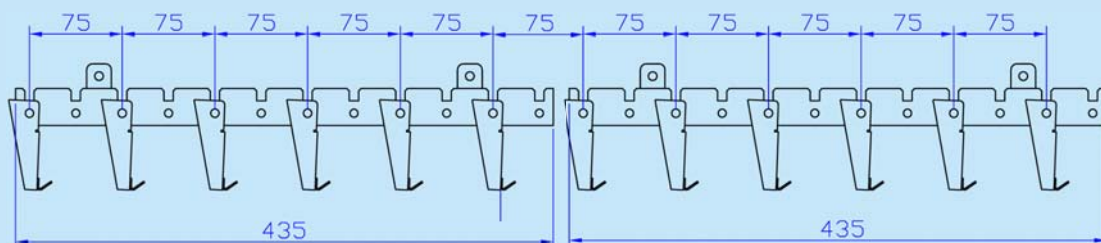
可選掛距2 Optional hanging spacing 2
