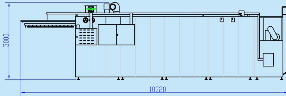
NS-395E-50 標準機型 Standard
