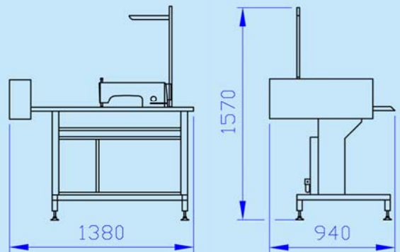
機身尺寸 Machine size
