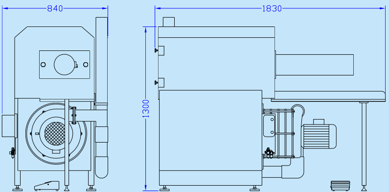
機身外形圖 Machine Size (mm)
