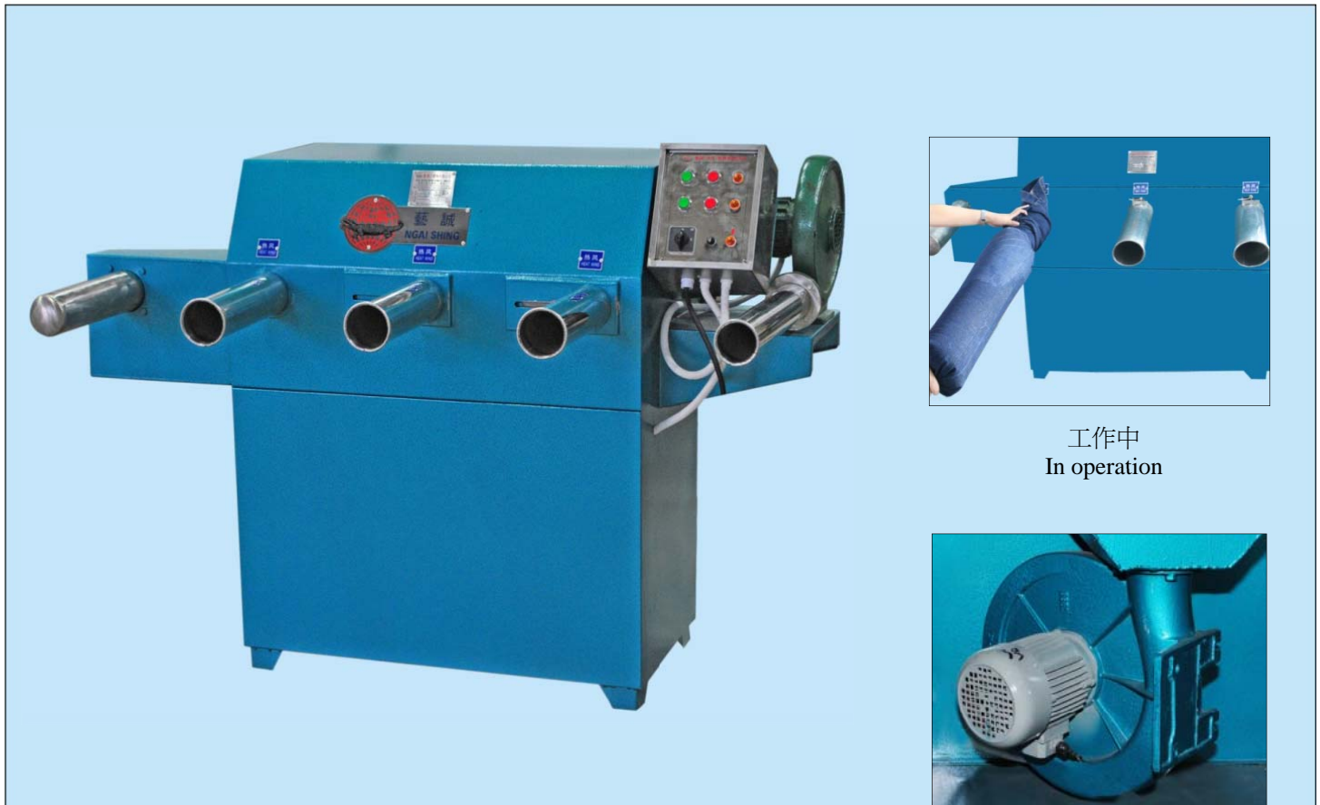
離心式中壓風機 Centrifugal medium pressure fan
