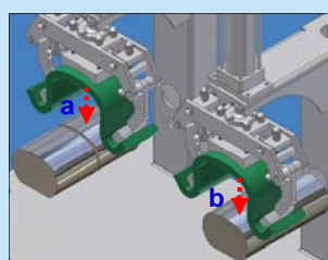
a. 熱壓狀態 Hot creasing b. 冷壓狀態 Cold creasing
