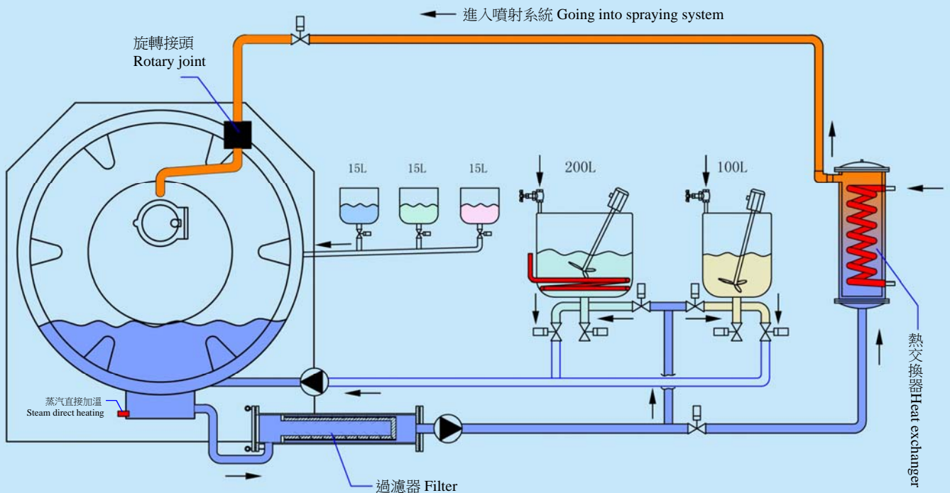
Farbe 360、Farbe 500工作原理圖 Working Principle
