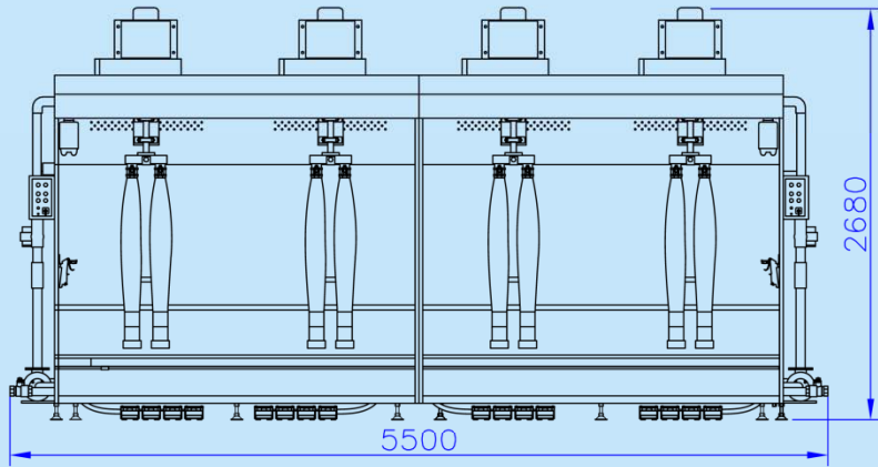
NS-8813A-50機身外形圖 Machine Size(Unit : mm)
