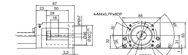
Motor Adaptor Flange F1
