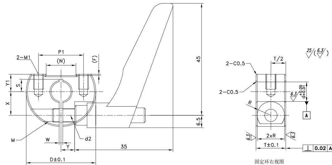
固定环右视图
